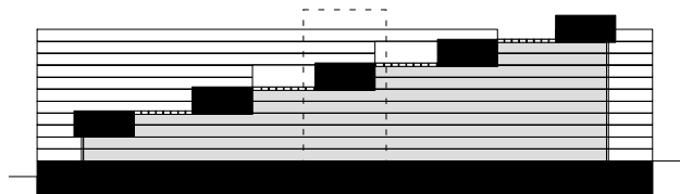
doorsnede atrium tussen oudbouw en nieuwbouw
